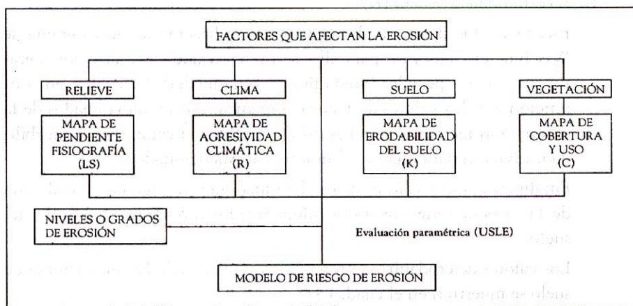
FIGURA 1 ESQUEMA GENERAL DE LA METODOLOGÍA PARA EL MAPEO DEL RIESGO DE EROSIÓN (SEGUN ALBADALEJO MONTORO)
